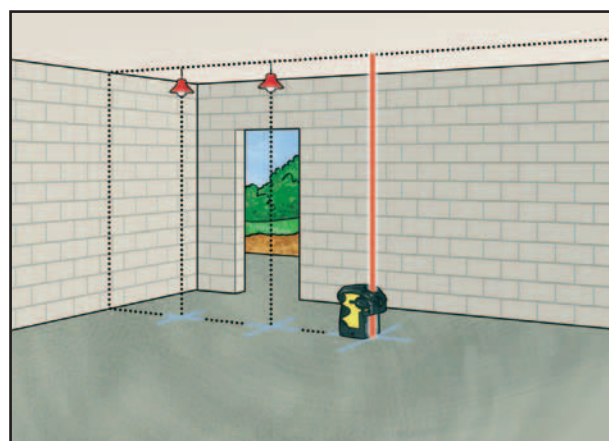
Přenášení bodů z podlahy na strop (případně naopak)
